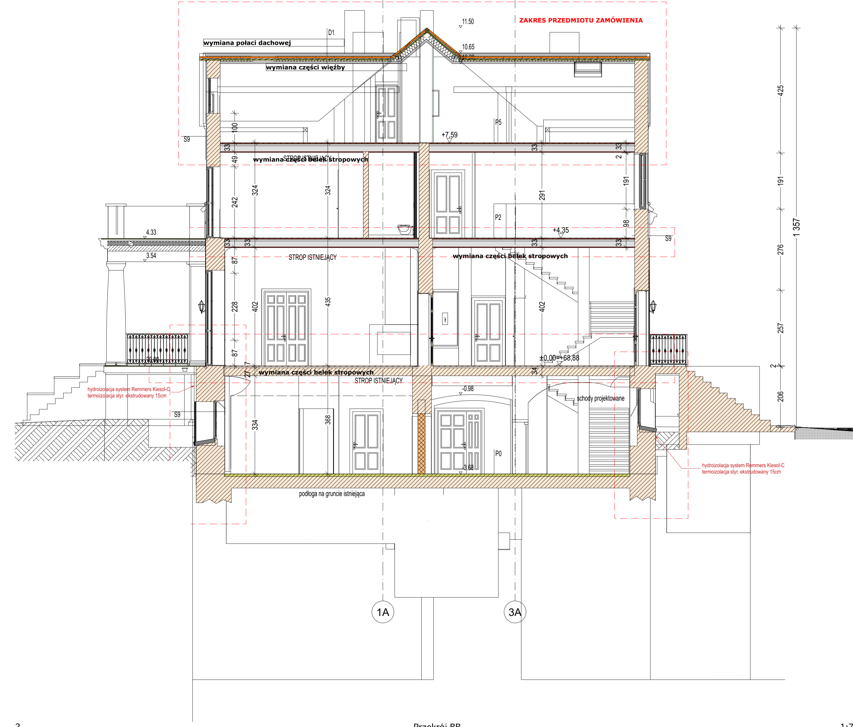
Przekrój BB
